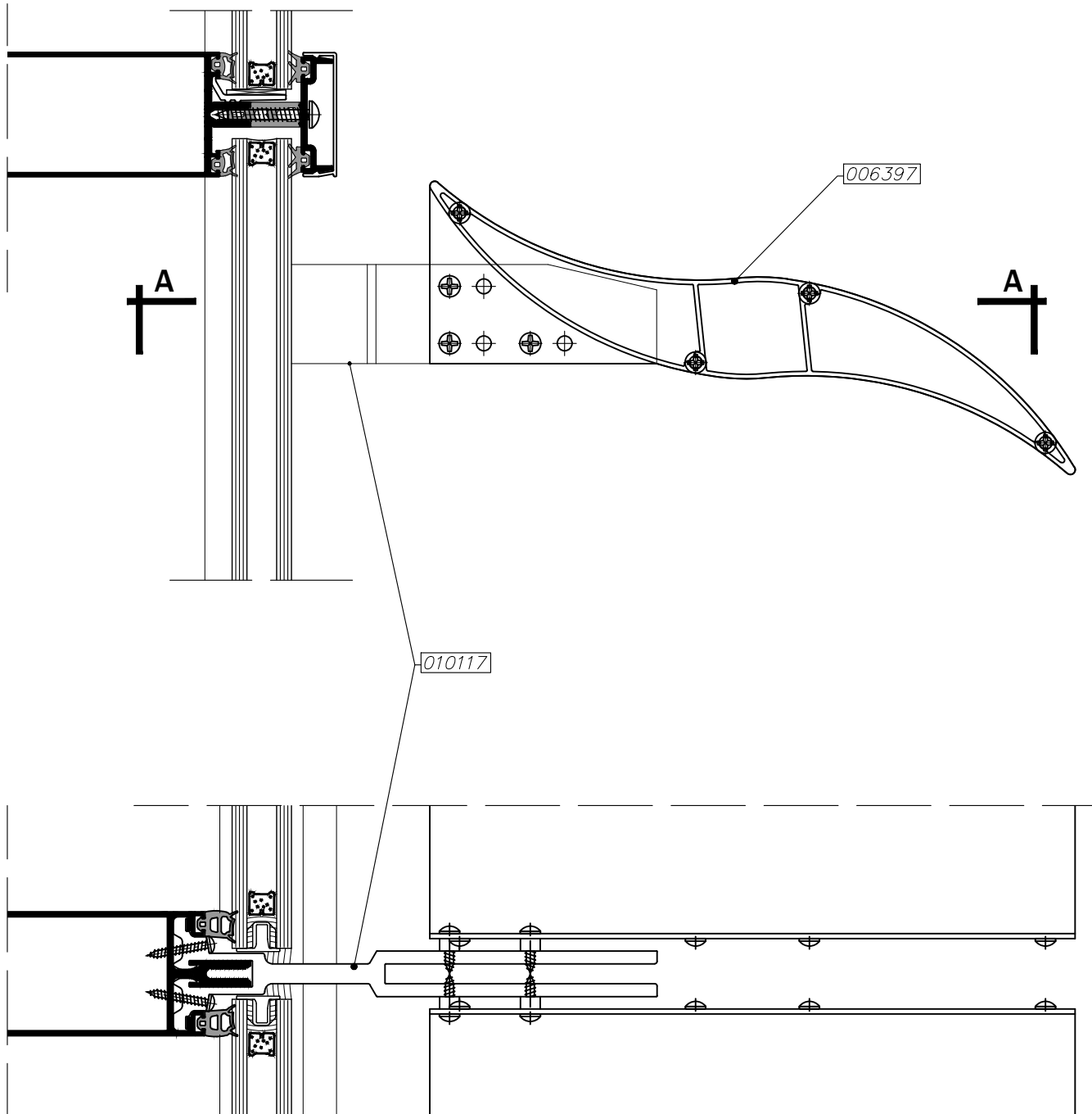
Section A-A
