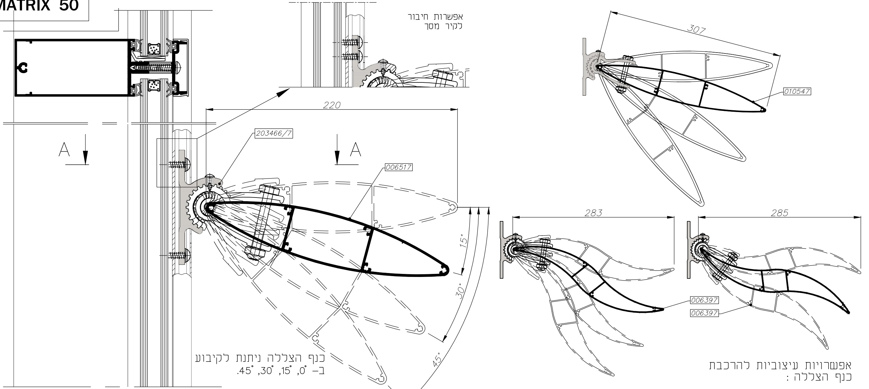
A-A פרט חיבור לקו רגולר
