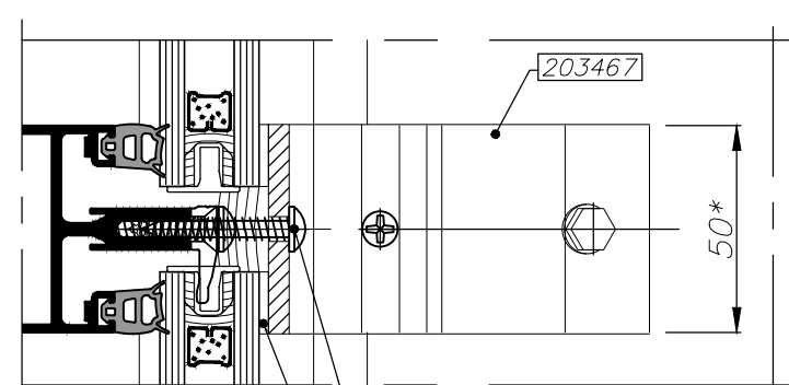
A-A פרט חיבור לקו סטרוקטורלי
