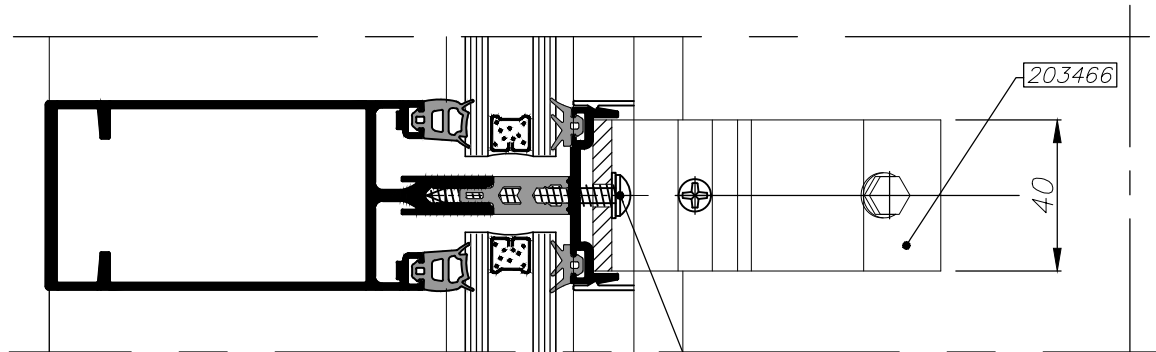
A-A פרט חיבור לקו רגולר
